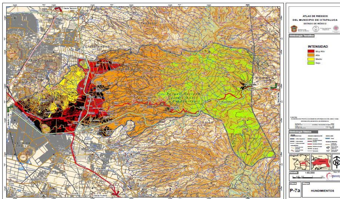
Mapa 11. Hundimientos en Ixtapaluca. Fuente: Atlas de Riesgo Municipal de Ixtapaluca 2018.
