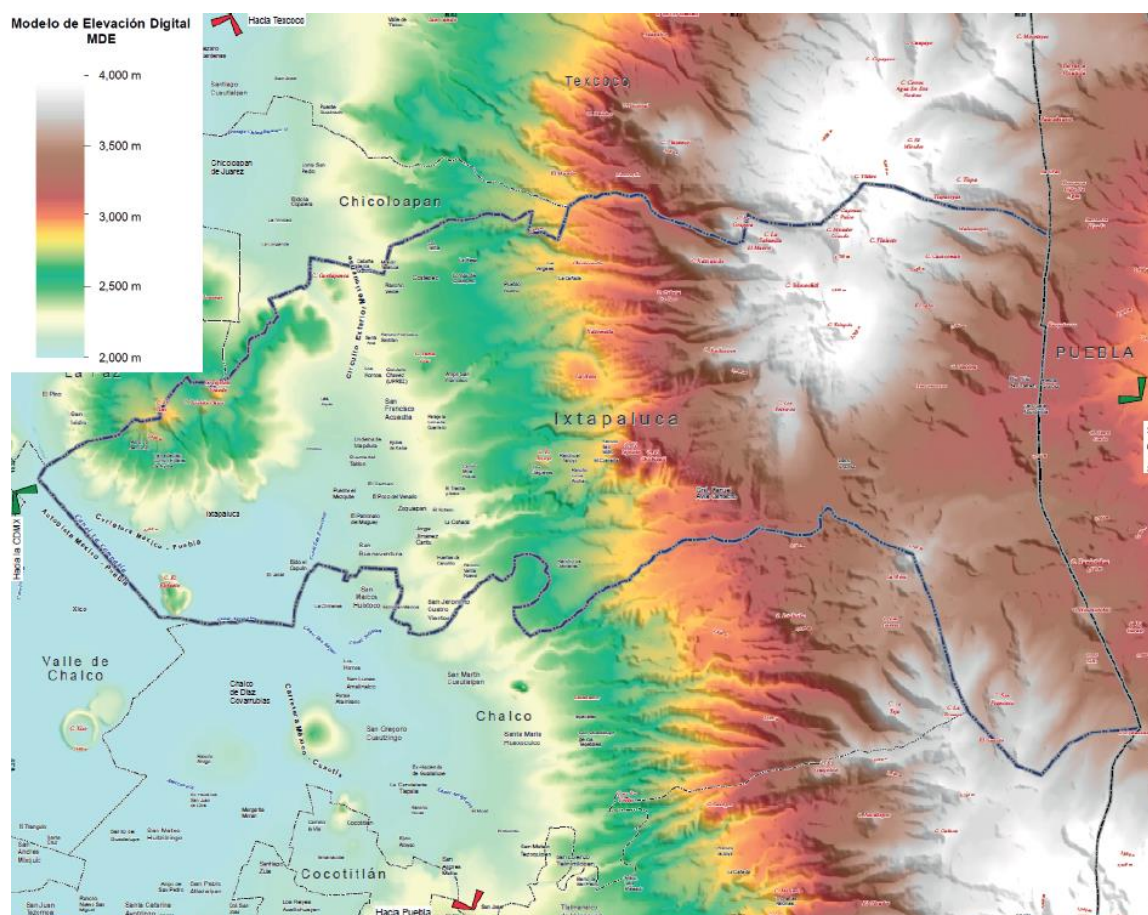
Mapa 5. Modelo de elevaciones del municipio de Ixtapaluca. Fuente: Elaboración propia con base en los datos de relieve del Continuo de elevaciones mexicano CEM (2.0) INEGI.
