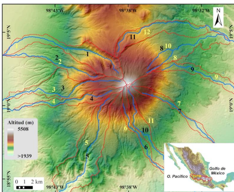
Imagen 22. Localización del Volcán Popocatepetl. Fuente: Boletín de la Sociedad Geológica Mexicana, UNAM, 2015.
