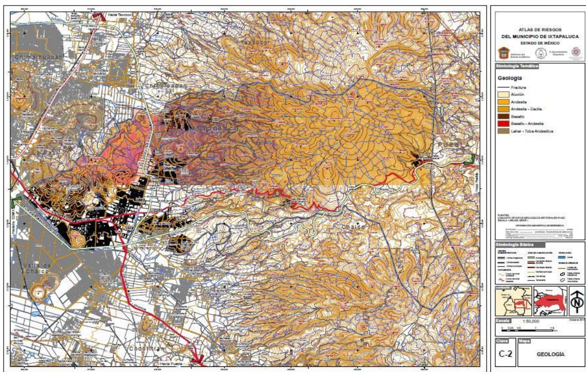
Mapa 10. Mapa geológico de Ixtapaluca. Fuente: Atlas de Riesgo Municipal de Ixtapaluca 2018.
